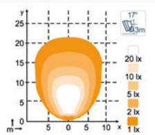
NORDIC LIGHTS CANIS PRO 330 3000 LM, 28 W.
